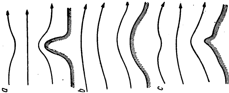
Rys. 74. Schemat przemieszczania się ku górze zaburzenia linii prądów wywołanego obecnością grzbietu górskiego w przypadku: a — wąskiego łańcucha górskiego, b — szerokiego łańcucha górskiego, c — szerokiego łańcucha górskiego z ostrą grania
