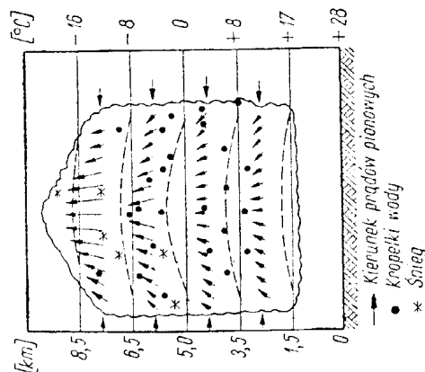
Rys. 67. Chmura w stadium rozwoju
