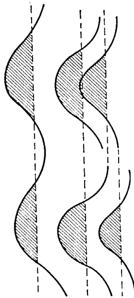
Rys. 88. Powstawanie chmur soczewkowatych kilkupiętrowych
