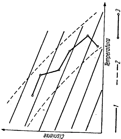
Rys. 33. Krzywa stratyfikacji 1 — adiabata sucha, 2 — adiabata wilgotna, 3 — krzywa stratyfikacji
