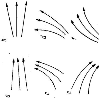
Rys. 15. Kształty linii prądów
