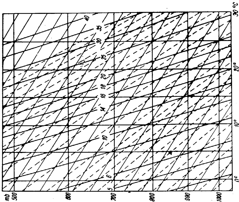
Rys. 31. Wycinek diagramu aerologicznego Linie poziome przedstawiają poziomy o jednakowym ciśnieniu, linie pionowe — izotermy, linie nachylone pod kątem 45° — suche adiabaty, linie kreskowane — adiabaty wilgotne, linie ciągłe lekko nachylone, opisane cyframi — izogramy
