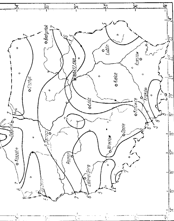
Rys. 120. Średni roczny procent dni z zachmurzeniem Cb nie dającym zjawisk burzowych, przy jednoczesnym występowaniu chmur niskich i średnich (typ C)
