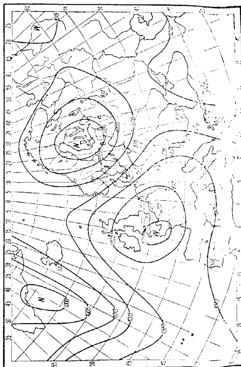
Rys. 99. Typ cyrkulacji C
