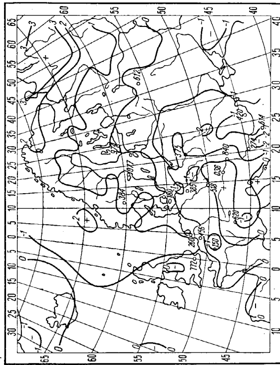
Rys. 25. Mapa tendencji ciśnienia z dnia 10.VI.1967 r.
