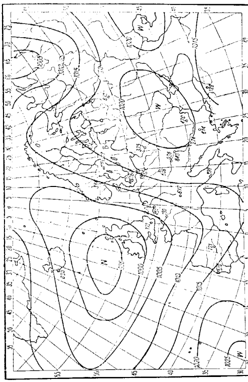
Rys. 105. Typ cyrkulacji E 1
