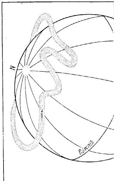
Rys. 90. Schemat jet-streamu na półkuli północnej
