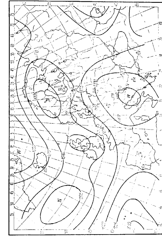
Rys. 103. Typ cyrkulacji D 2 C
