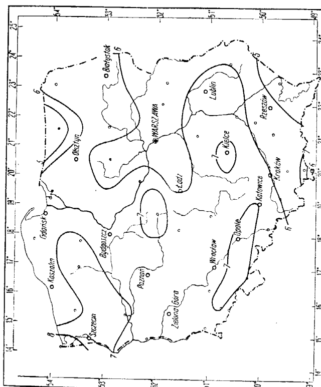
Rys. 119. Średni roczny procent dni z zachmurzeniem Cu cong przy jednoczesnym występowaniu chmur niskich i wysokich (typ B_2 )
