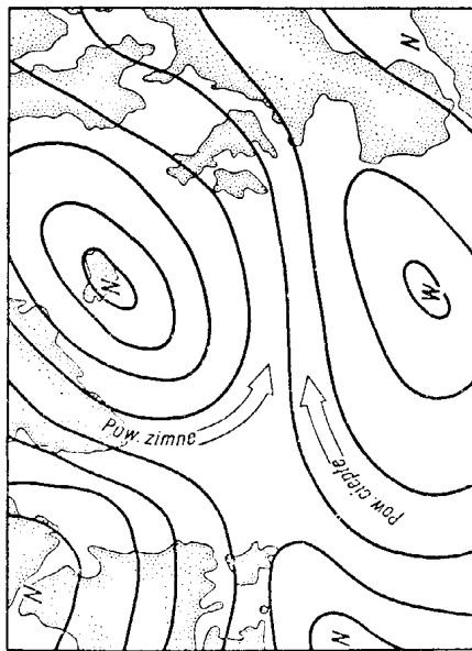
Rys. 91. Schematyczna sytuacja pogotowa sprzyjająca rozwojowi jet-streamu w obszarze atlantycko-europejskim
