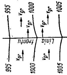
Rys. 10. Front prostopadły do izobar; front taki przemieszcza się w kierunku i z prędkością wiatru gradientowego
