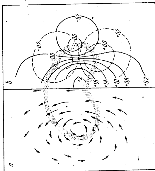
Rys. 51. Schemat odizolowanego pęczera ciepłego powietrza - - - - - prędkości poziome, ——— izotachy prądów wstępujących
