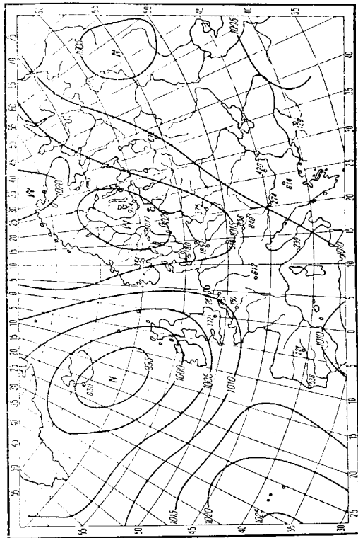
Rys. 104. Typ cyrkulacji E
