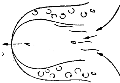
Rys. 39. Schemat pęcherza termicznego
