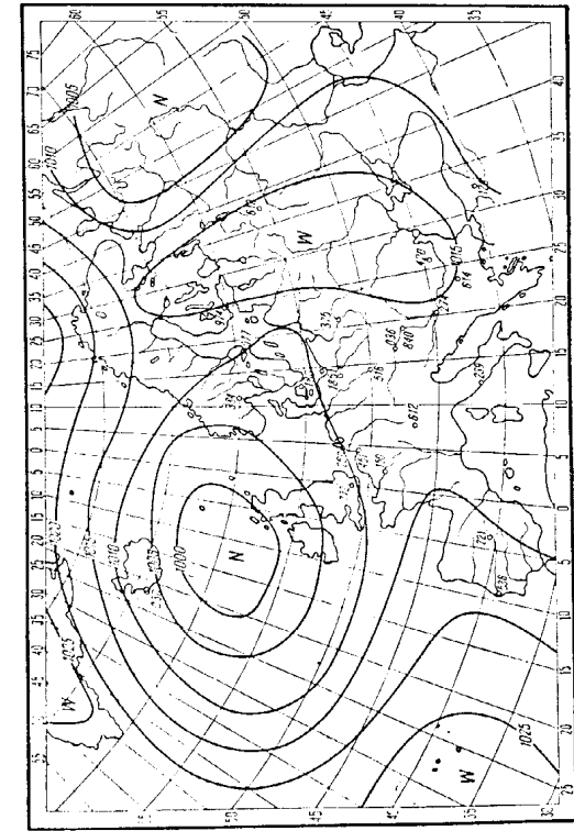
Rys. 102. Typ cyrkulacji D
