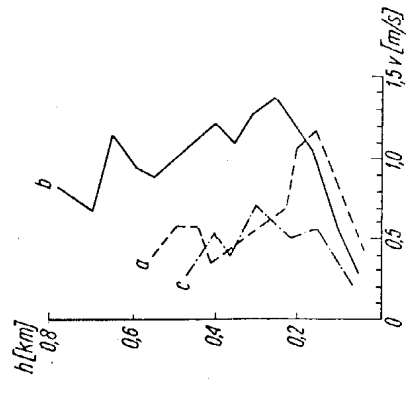
Rys. 61. Rozkład średnich prędkości prądów wstępujących w zależności od pory dnia przy termie cumulusowej a — przed południem, b — w południe, c — po południu
