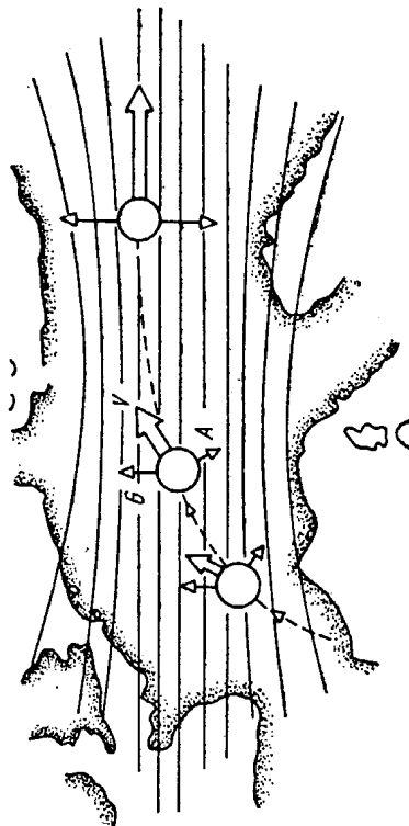
Rys. 13. Działanie siły Coriolisa na cząstkę powietrza
