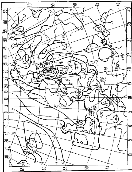
Rys. 23. Mapa tendencji ciśnienia z dnia 8.VI.1967 r.
