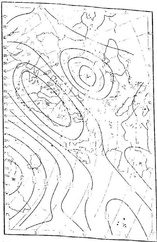
Rys. 107. Typ cyrkulacji E_1
