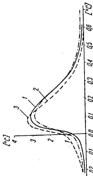
Rys. 48. Rozkład prądów konwekcyjnych w zależności od temperatury 1 — rano, 2 — w południe, 3 — wieczorem oś pozioma — różnice temperatur pomiędzy powietrzem otaczającym a średnią temperaturą komina, oś pionowa — temperatura różnienia komina
