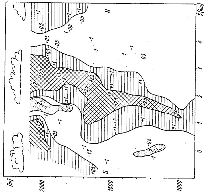
Rys. 54. Pionowy przekrój przez komin termiczny pod podstawą Cubum
