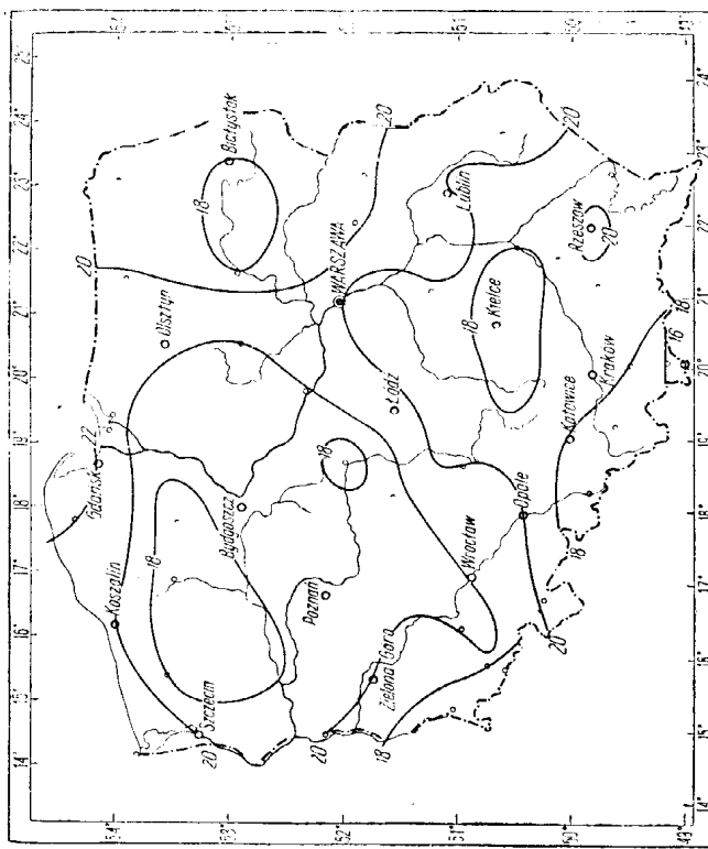
Rys. 115. Średnia liczba dni z zachmurzeniem konwekcyjnym we wrześniu
