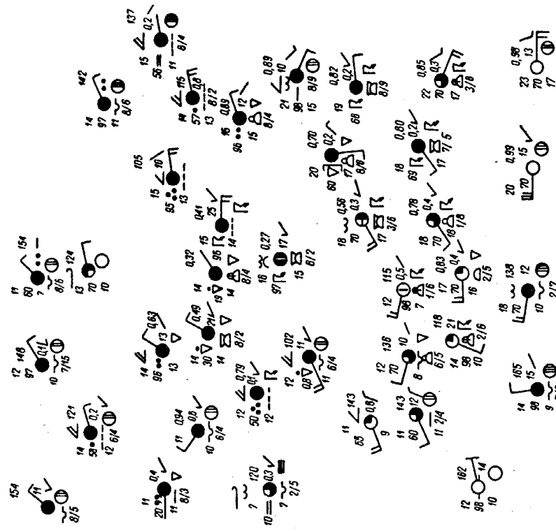
Rys. 18. Wycinek mapy synoptycznej z naniesionymi danymi — nieprzeanalizowany
