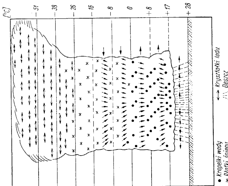
Rys. 70. Chmura burzowa w stadium rozpada
