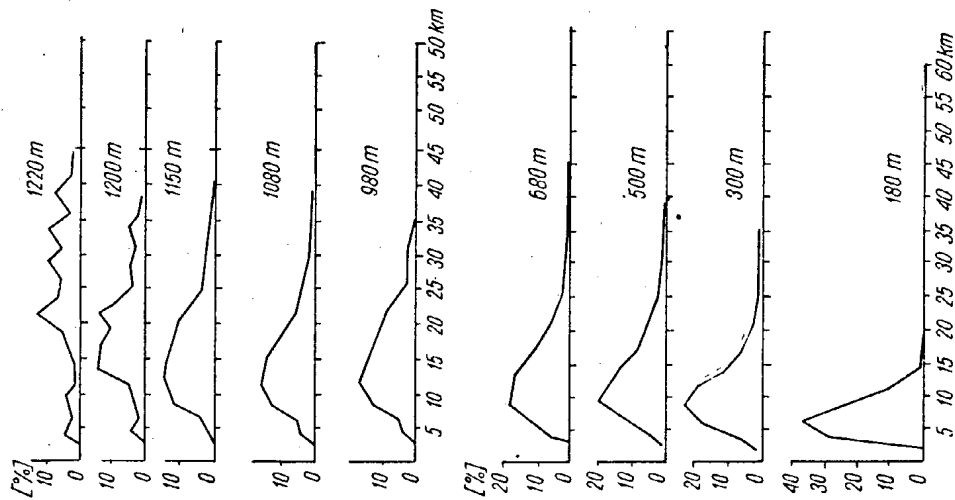
Rys. 63. Krzywe rozkładu częstości (%) średnic kropli w chmurach kłębiastych w zależności od wysokości
