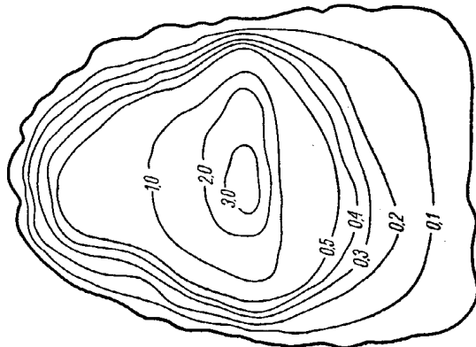
Rys. 65. Wodność chmury kłębiastej ( \text{g/m}^3 ) (Rozkład wodności z pomiaru dokonanego przez Zajcewa 23.VII.1949 r.)
