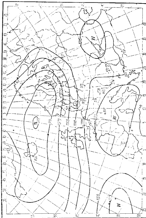
Rys. 97. Typ cyrkulacji A
