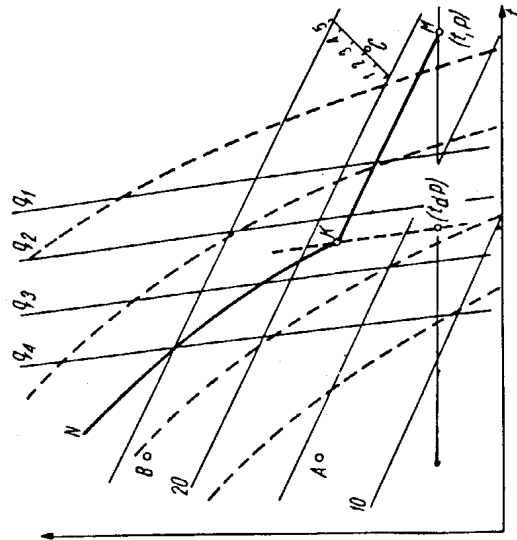
Rys. 35. Krzywa stanu MKN — krzywa stanu, q_1, q_2, q_3, q_4 — izogramy, K — punkt kondensacji
