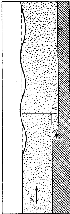
Rys. 73. Zaburzenia falowe na powierzchni wody przez lokalne zwiększenie głębokości strugi
