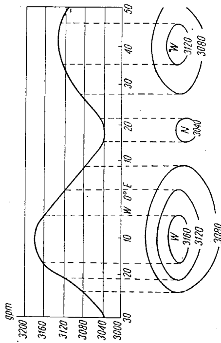
Rys. 29. Przekrój pionowy (u góry) i mapa topografii bezwzględnej (na dole skonstruowane na podstawie mapy TB_{700} z dnia 10.VI.1967 r.; przekrój wykonany wzdłuż 50^{\circ}N na odcinku 30^{\circ}W - 50^{\circ}E
