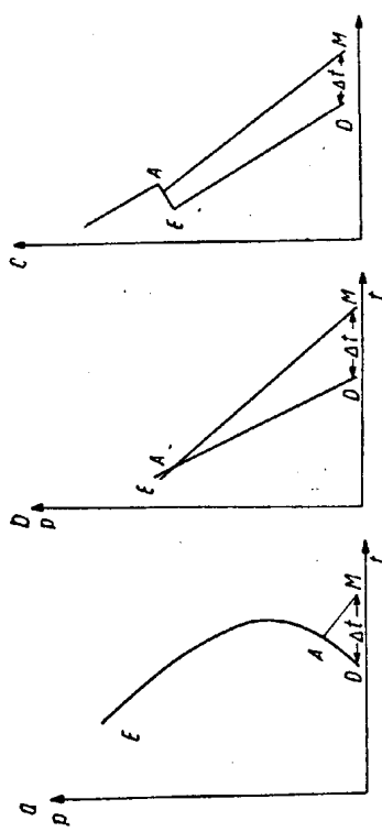
Rys. 36. Określanie poziomu konwekcji „suchej”
