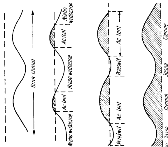
Rys. 87. Powstawanie chmur soczewkowych przy różnej wilgotności względnej powietrza — — — — — poziom kondensacji powietrza wznoszącego się
