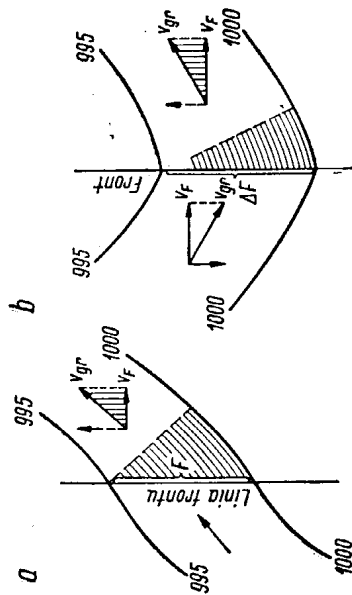
Rys. 11. Front przecinający izobary pod kątem ostrym; przesuwa się on w kierunku i z prędkością składowej wiatru gradientowego prostopadłej do frontu
