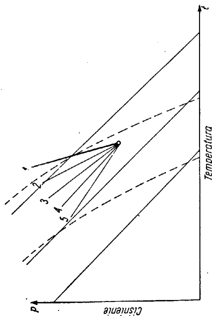
Rys. 32. Graficzne określenie równowagi pionowej
