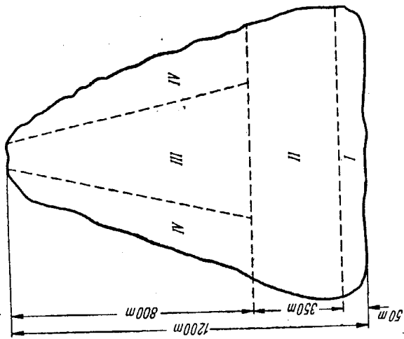
Rys. 64. Schemat rozkładu kropli w chmurze kłębiastej
