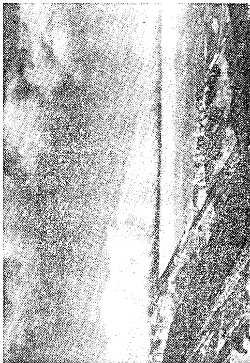
Rys. 86. Mur halny w Skalnym Pleso w Tatrach Słowackich
