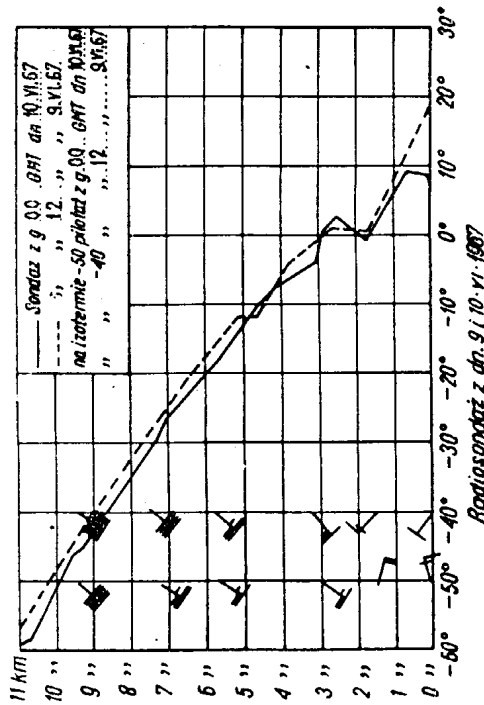
Rys. 26. Radiosondaż z dnia 9 i 10.VI.1967 r.
