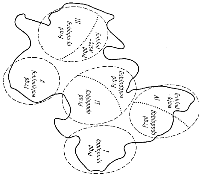
Rys. 71. Poziomy przekrój przez skupisko chmur burzowych (I ÷ V)
