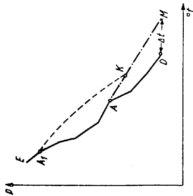
Rys. 37. Określanie poziomu konwekcji „wilgotnej”
